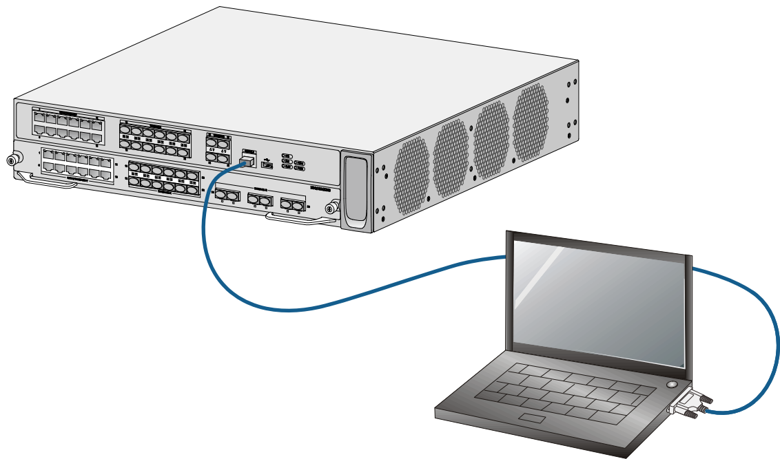
图4-1 连接配置口电缆
