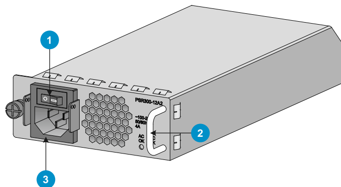
图A-4 交流电源模块外观
