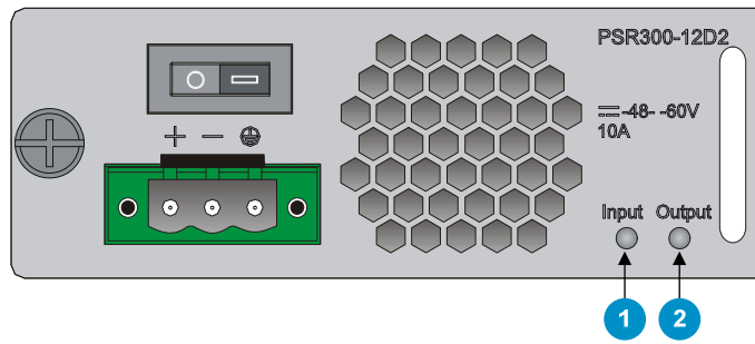
图B-2 直流电源指示灯
