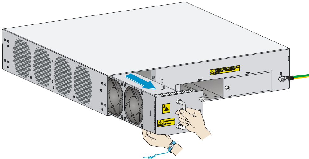
图5-5 将风扇框拉出风扇框插槽
