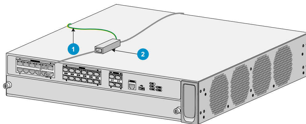
图3-11 网口避雷器安装示意图
