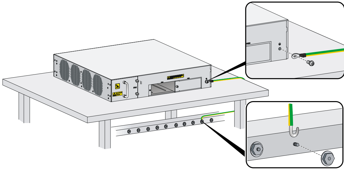
图3-7 通过接地排接地.
