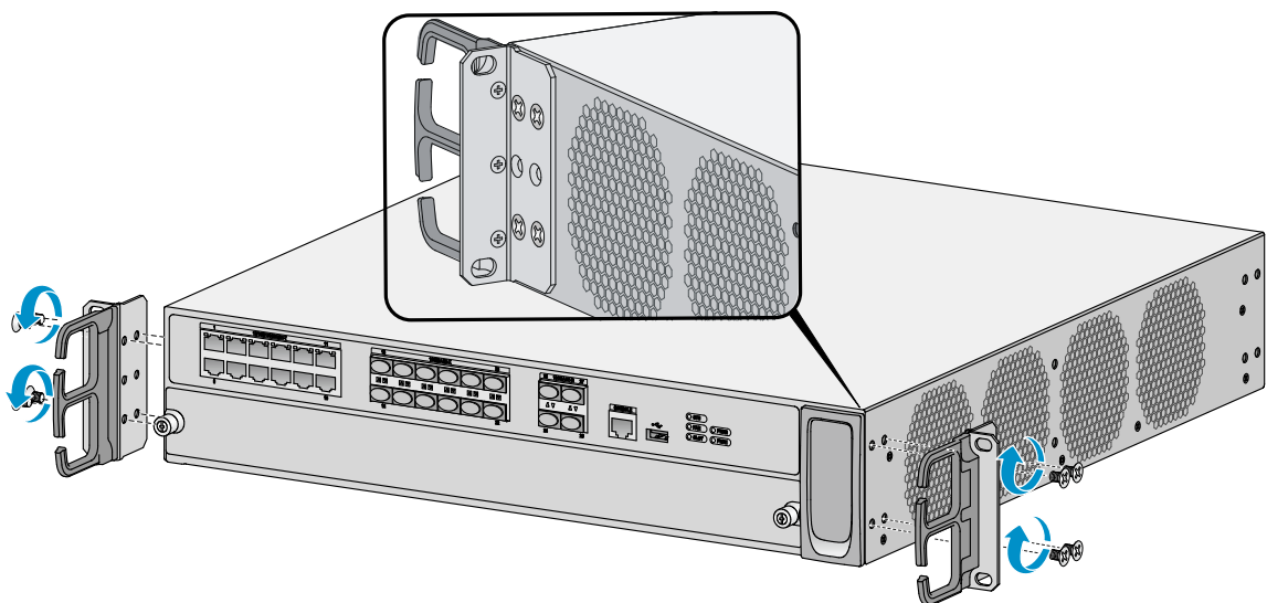
图3-4 安装挂耳到设备前面板的左、右两侧
