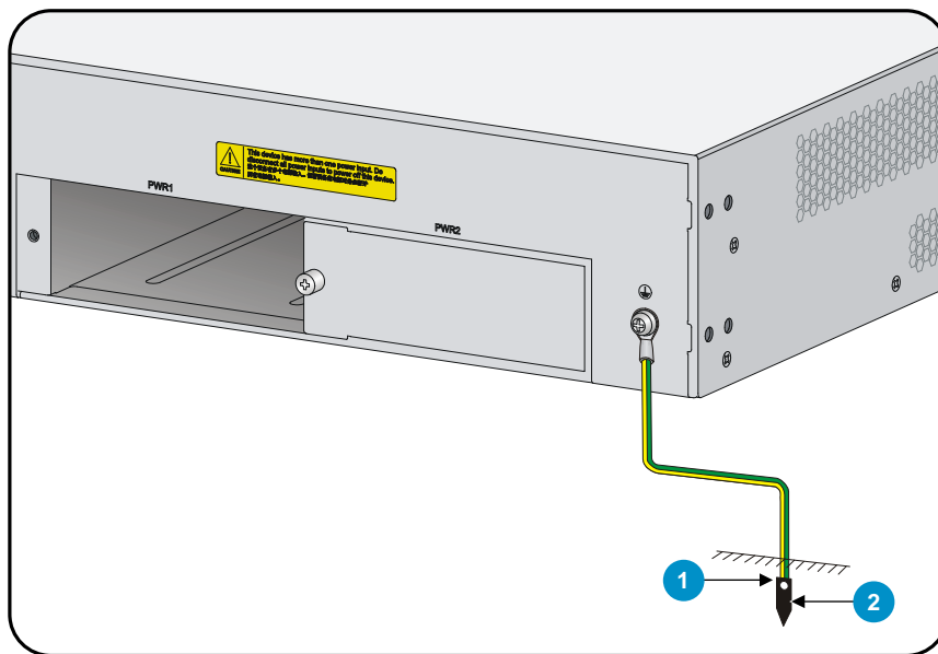
图3-8 机房附近允许埋设接地体时接地安装简图
