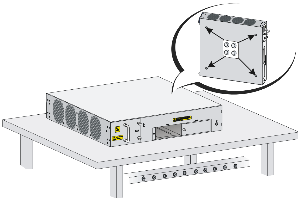
图3-2 工作台安装方式
