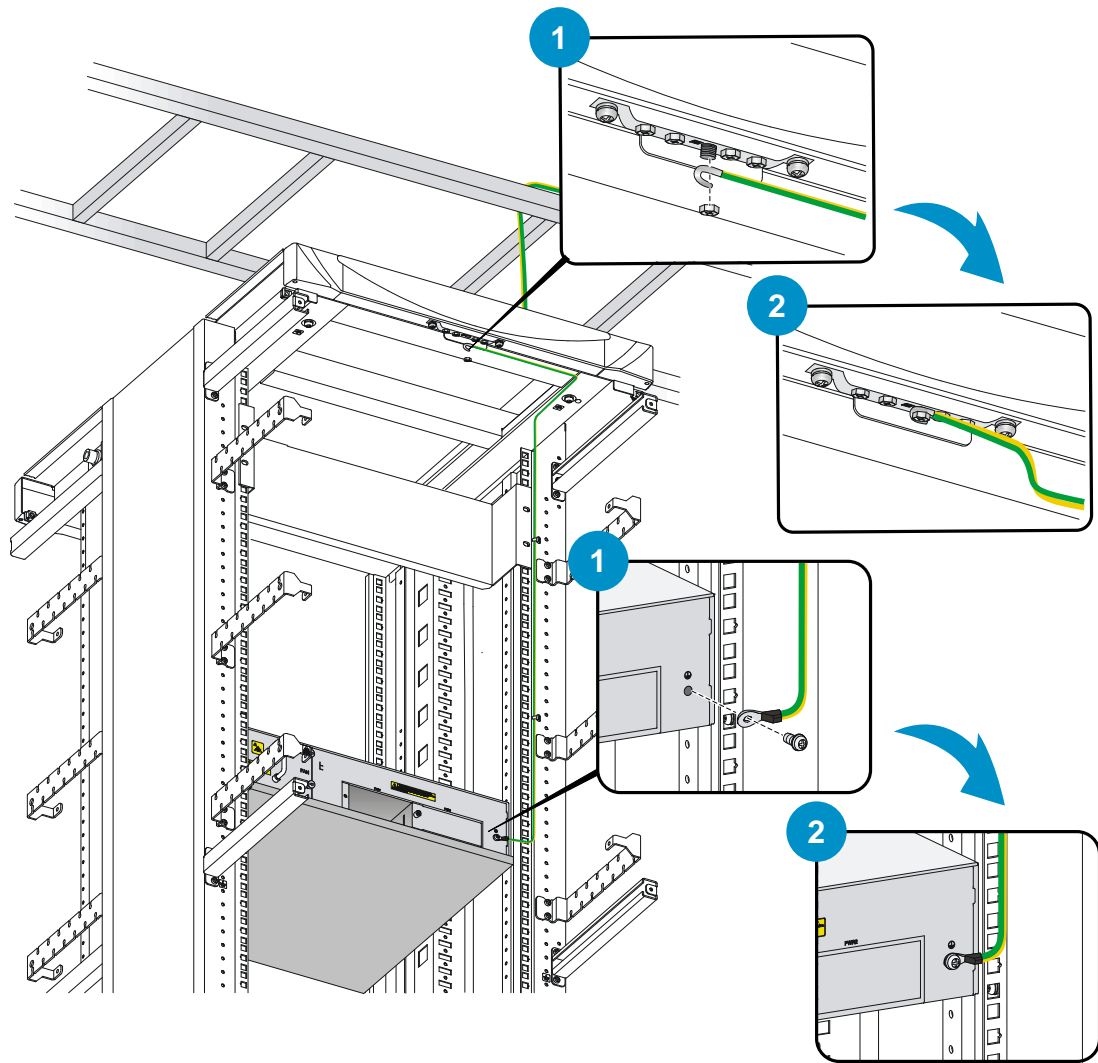
图3-6 连接到机柜接地
