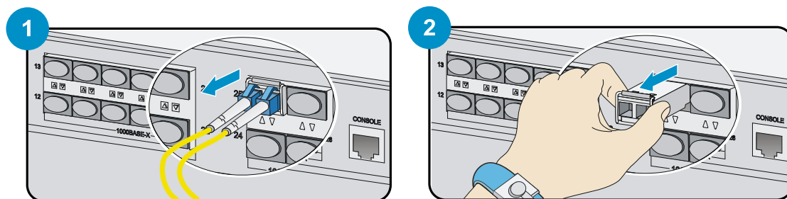
图5-4 拆卸光接口模块示意图
