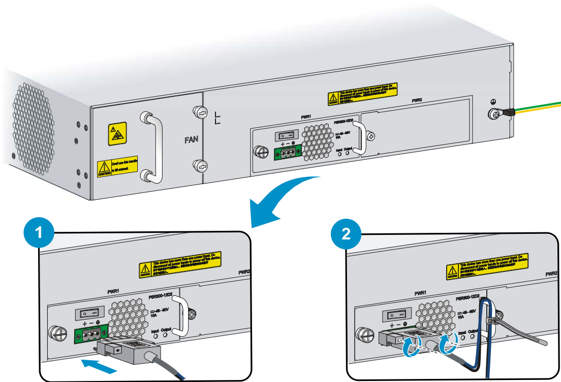
图3-17 连接直流电源线
