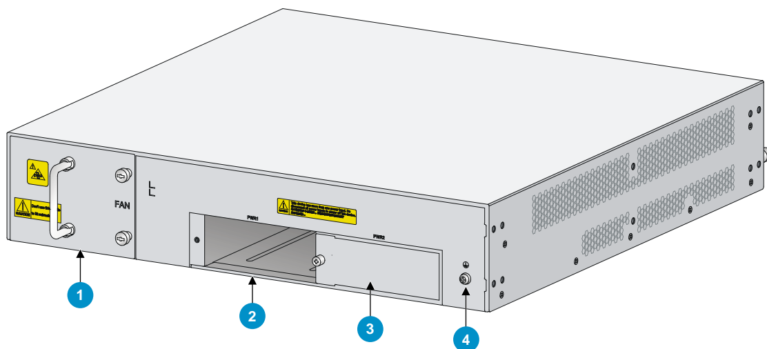
图A-2 设备后视图
