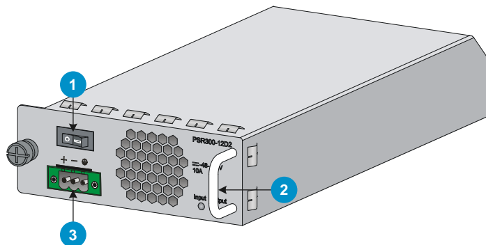
图A-5 直流电源模块外观
