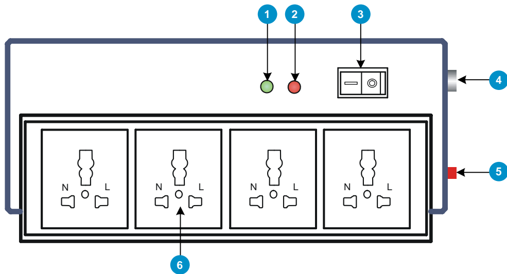
图3-12 电源避雷器示意图
