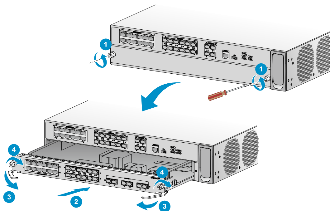
图3-10 安装 NSQ1G24XS60 接口板
