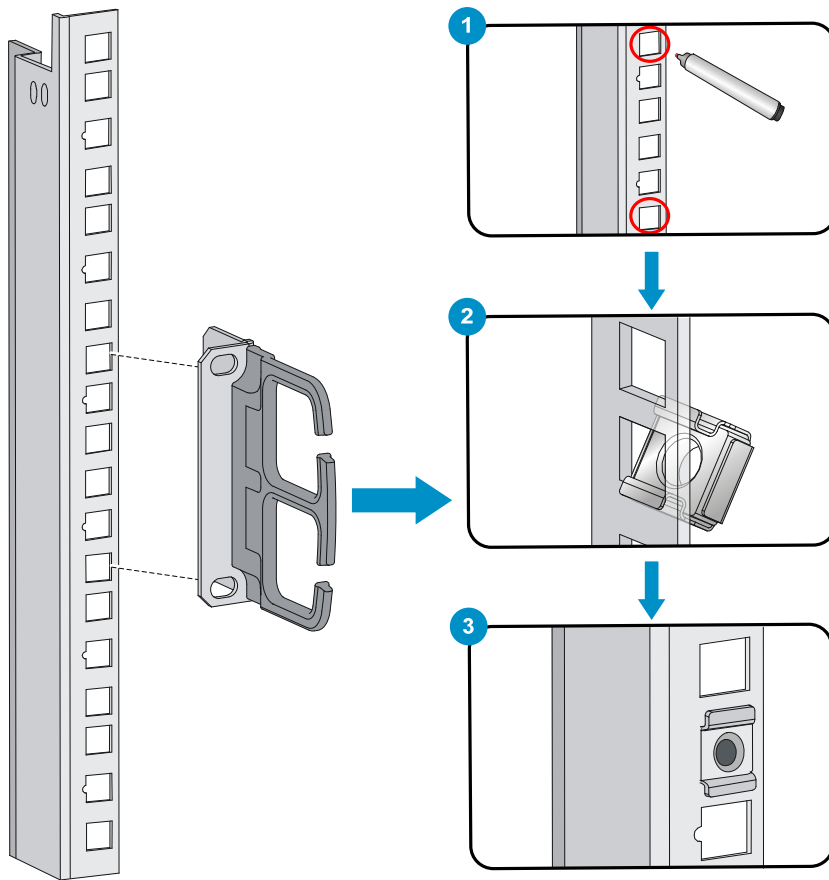
图3-3 安装浮动螺母
