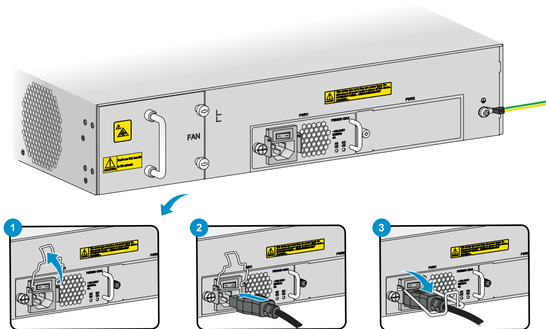
图3-16 连接交流电源线
