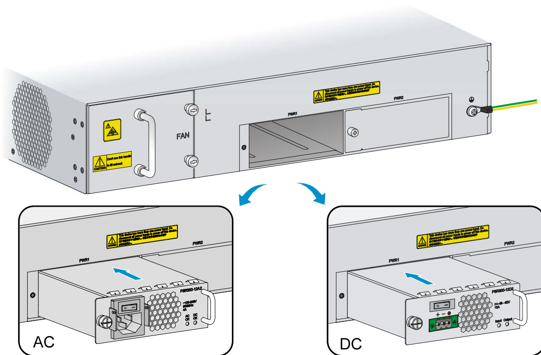
图3-9 安装电源模块
