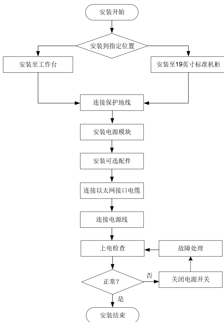
图3-1 设备安装流程示意图
