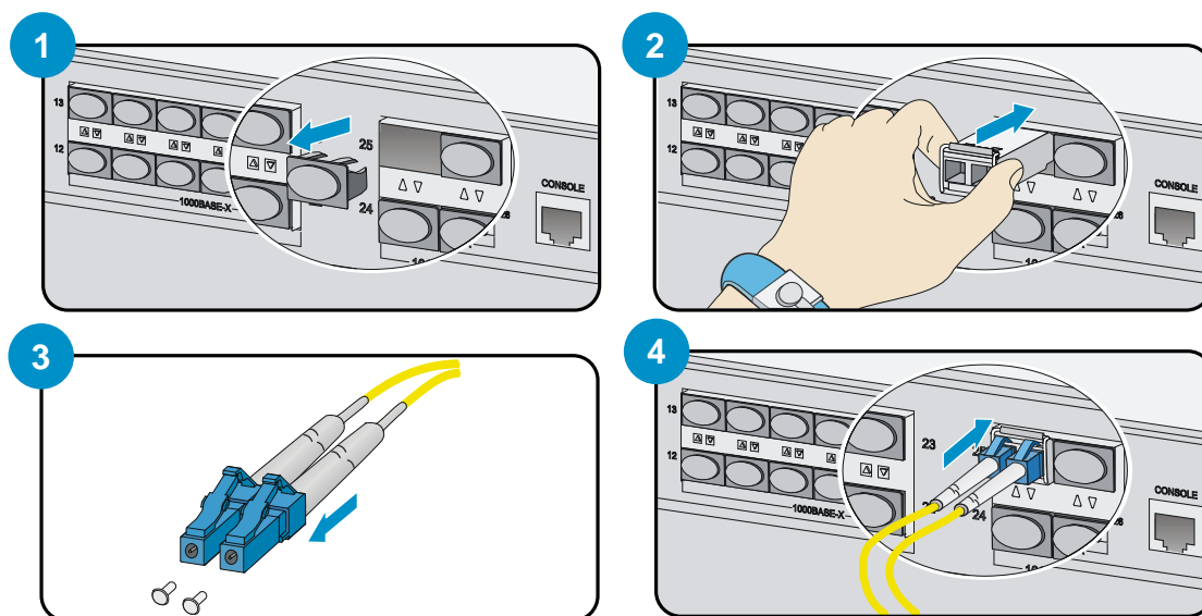
图3-15 连接光纤
