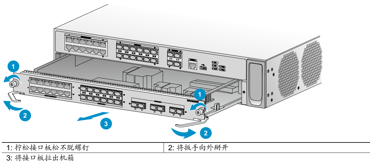
图5-2 拆卸 NSQ1G24XS60 接口板
