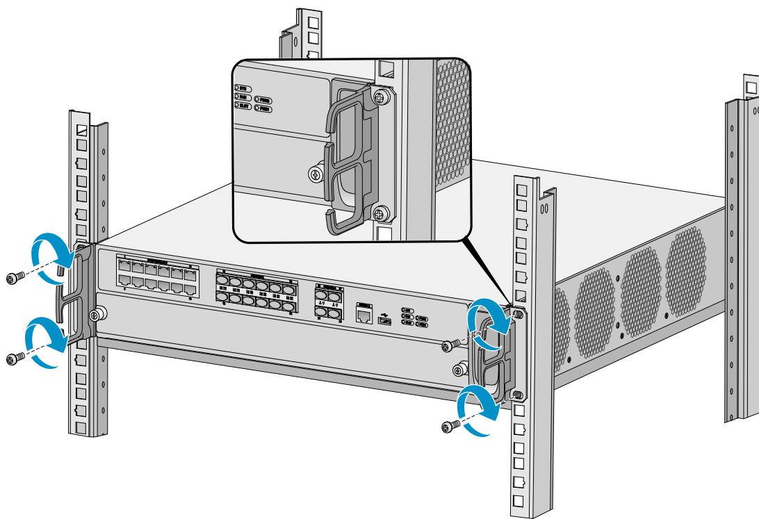
图3-5 安装设备到机柜
