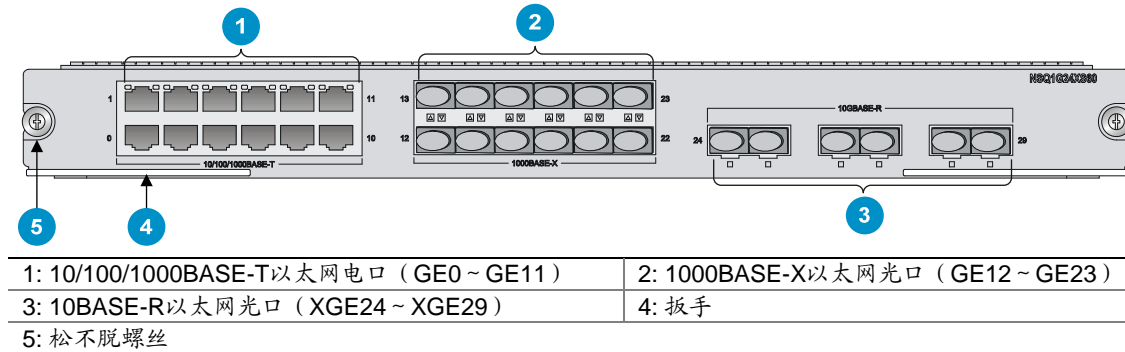
图A-3 NSQ1G24XS60 接口板正视图
