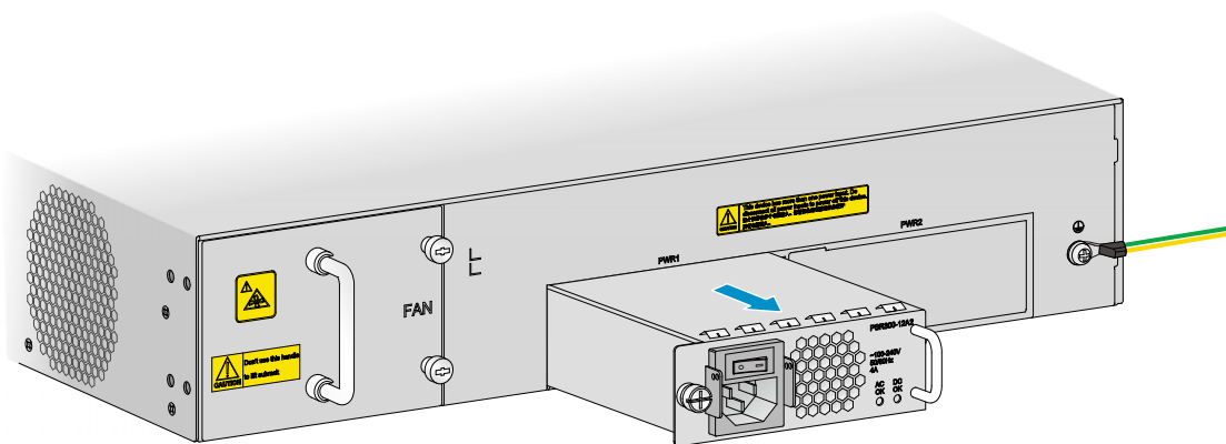
图5-1 拆卸电源模块
